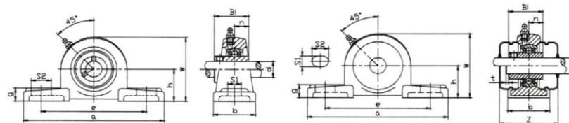
UCP200 SERIES UCP200 系列
