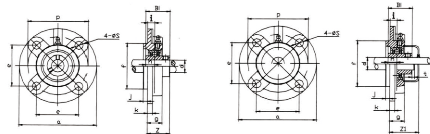
UCFC200 SERIES UCFC200 系列
