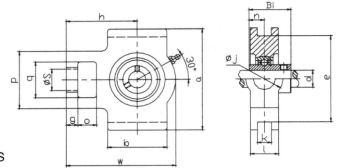
UCT300 SERIES UCT300 系列
