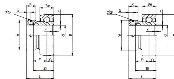
SA200 SERIES SA200 系列
