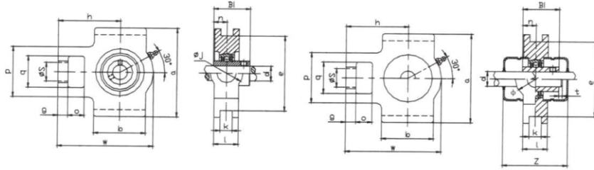
UCT200 SERIES UCT200 系列
